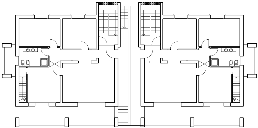
P RIALZATO
