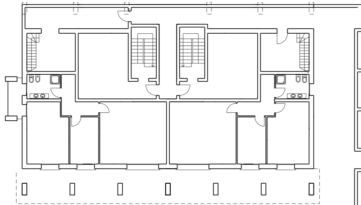
P SEMINTERRATO
