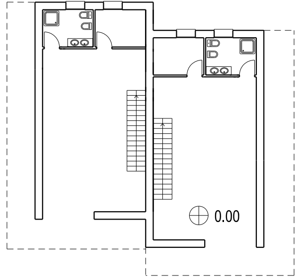
P SEMINTERRATO
