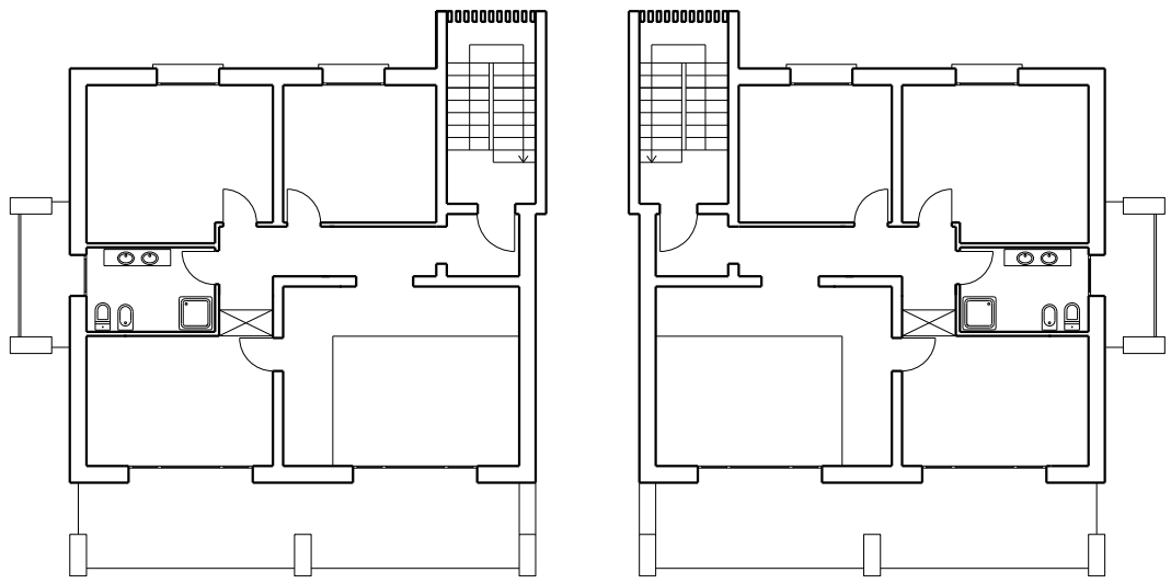
P PRIMO
