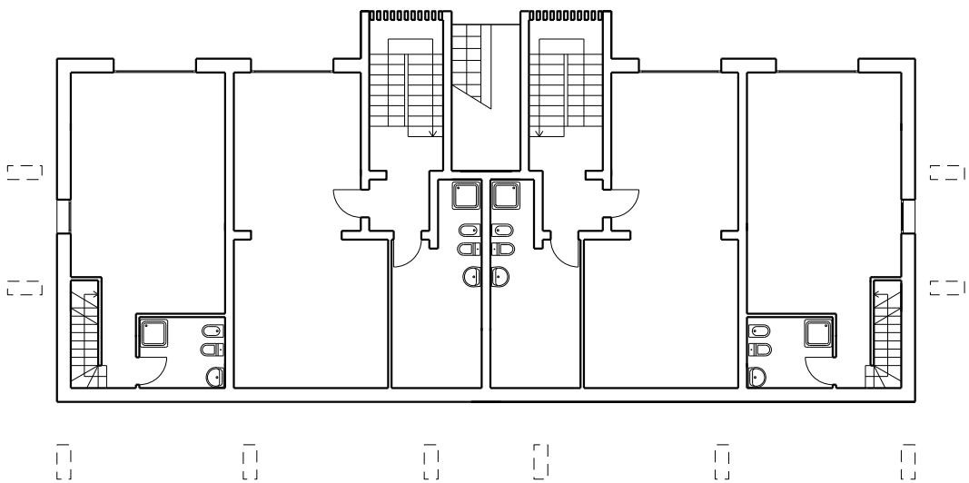
P SEMINTERRATO
