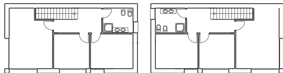
P SEMINTERRATO 2
